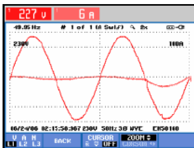
Фазное напряжение и ток обходной линии ИБП, "красная" фаза
